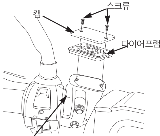
마스터실린더 보디
