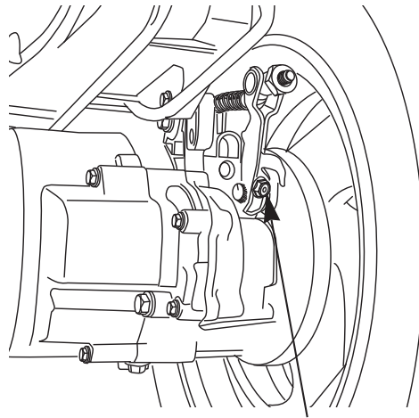
브레이크암 인디케이트
