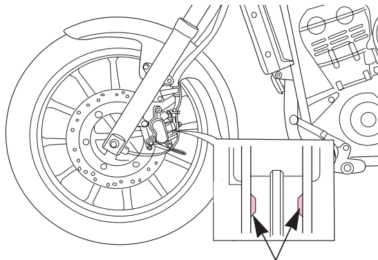
마모한계선
