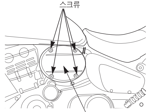
에어 크리너 케이스커버
