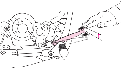
(브레이크페달의 유격)
