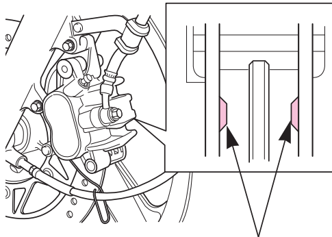
마모한계선
