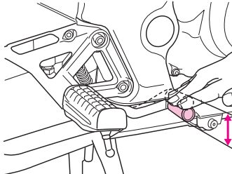
(브레이크페달의 유격)
