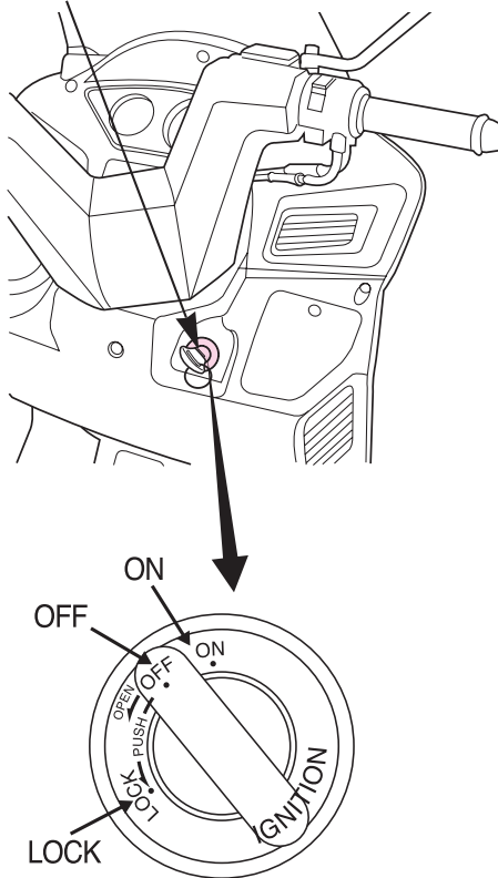
메인 스위치
