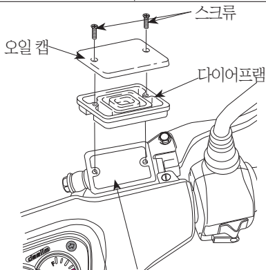
마스터실린더 보디
