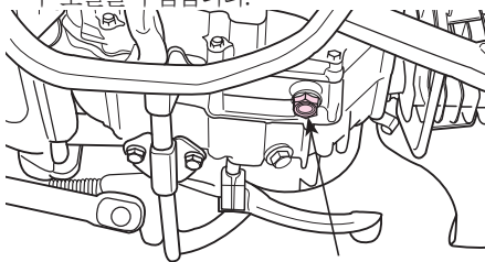
드레인 플러그
