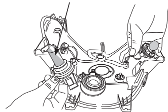
헤드라이트 벌브
