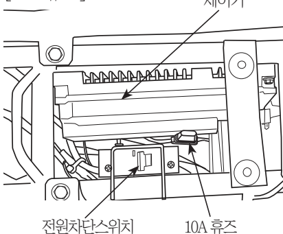
[ 10A 휴즈 ]
