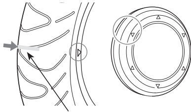
웨어인디케이터위치 표시마크
